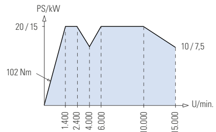
Spindelkasten 15.000 U/min. – Dauerbetrieb S1
