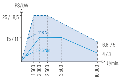
Spindelkasten 10.000 U/min. – Interimsbetrieb S3-15%
